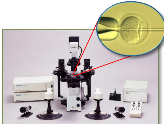
↑ PMM付マイクロマニピュレーションシステムの一般的な構成 (丸抜き)マウス核移植操作画像 【XenoWorks PT】
